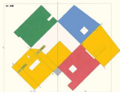
折り紙建築による外皮(八代克彦)
