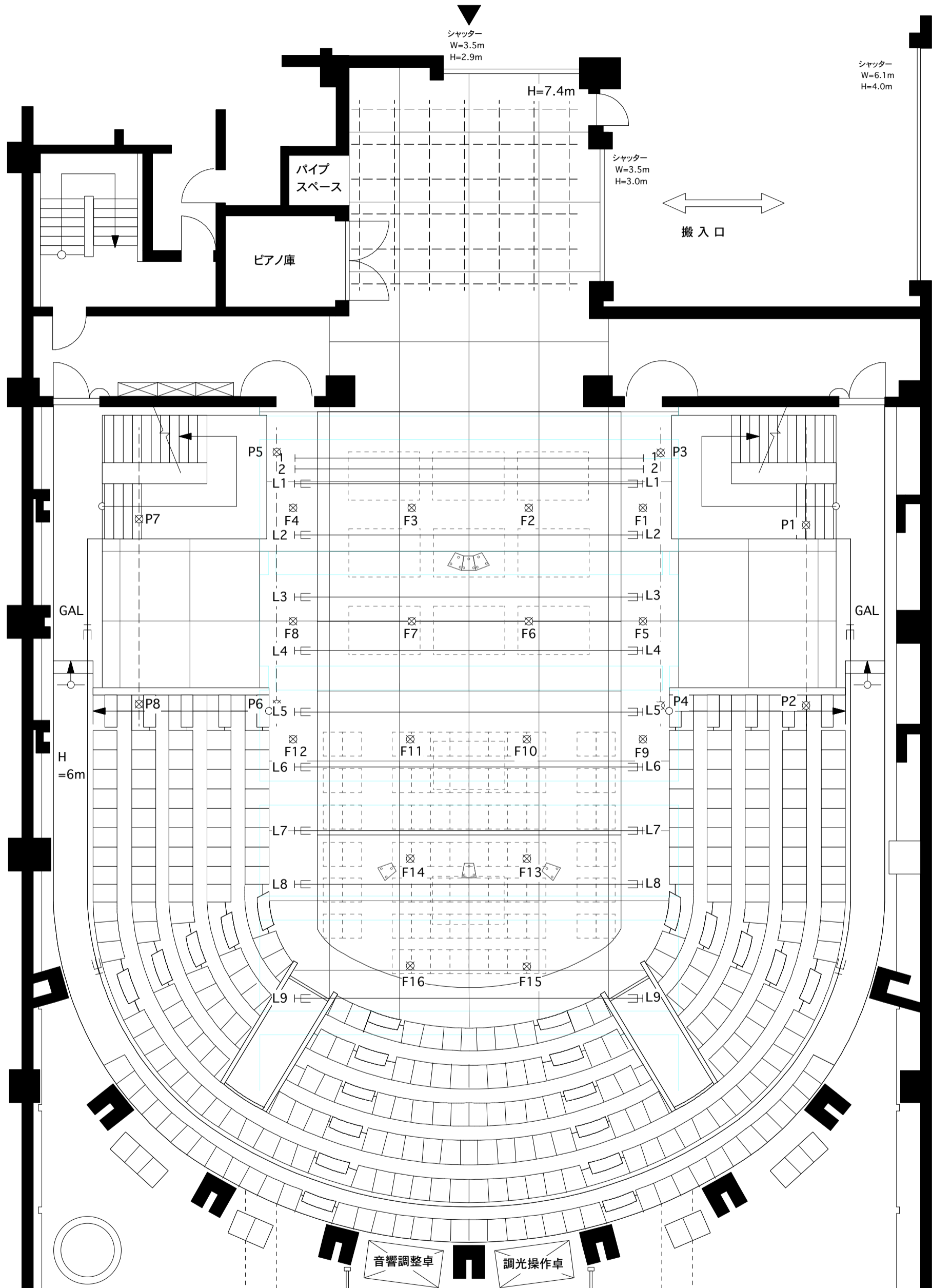
彩の国さいたま芸術劇場 小ホール 舞台平面図 S=1:100
